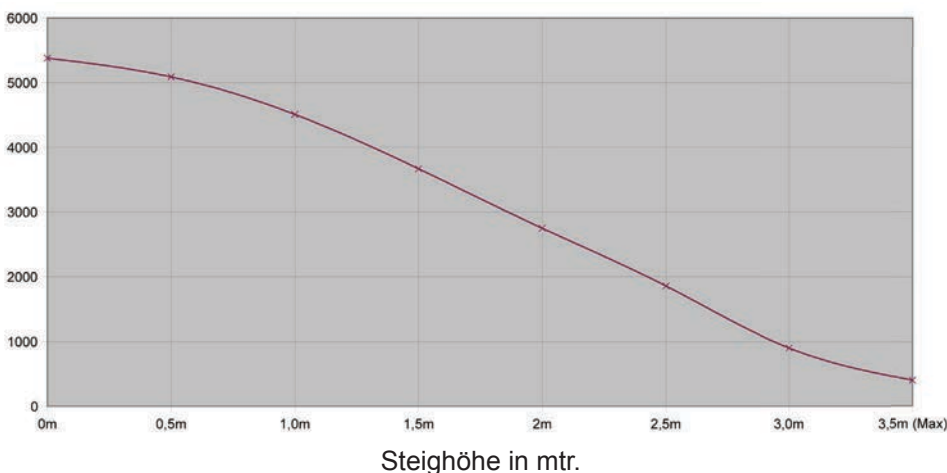
Liter/h Leistungskurve bei 50W Vollast
