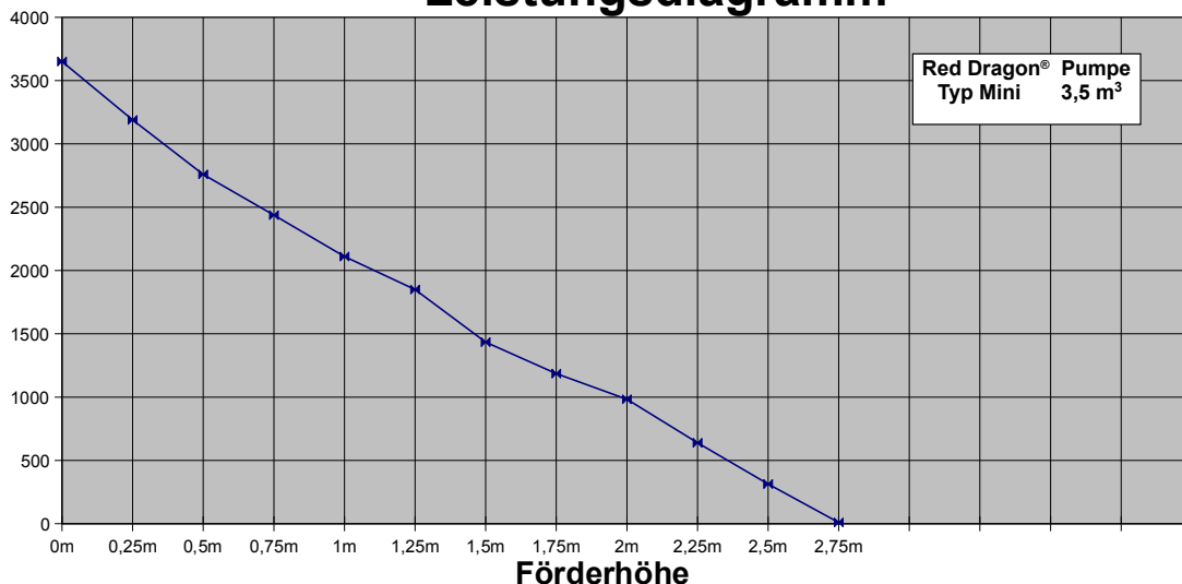
Liter / h Leistungsdiagramm
